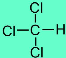
Chloroform
